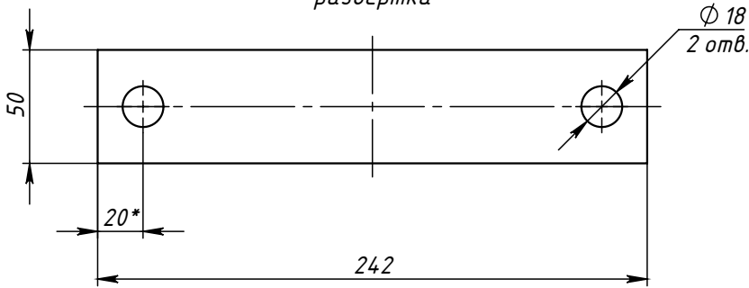
Поз.2 (Полухомут) развертка
